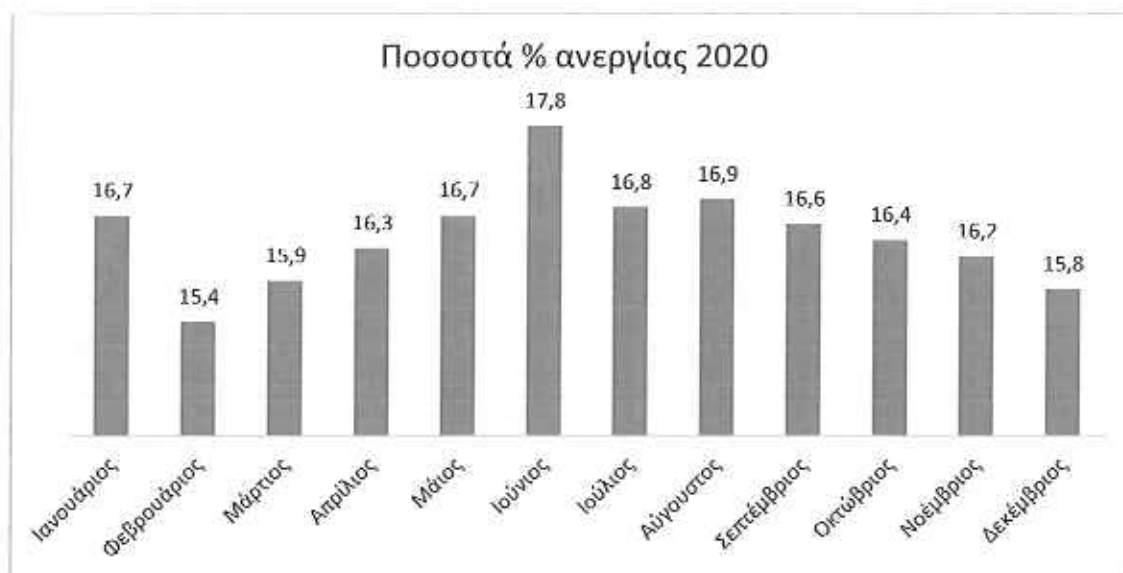
ΠΙΝΑΚΑΣ-ΓΡΑΦΗΜΑ 1: ΠΟΣΟΣΤΟ ΑΝΕΡΓΙΑΣ ΑΝΑ ΜΗΝΑ ΤΟΥ ΕΤΟΥΣ 2020
